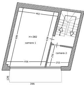
PIANO SECONDO
