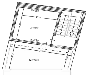
PIANO SOTTOTETTO
