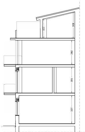
SEZIONE A-A
